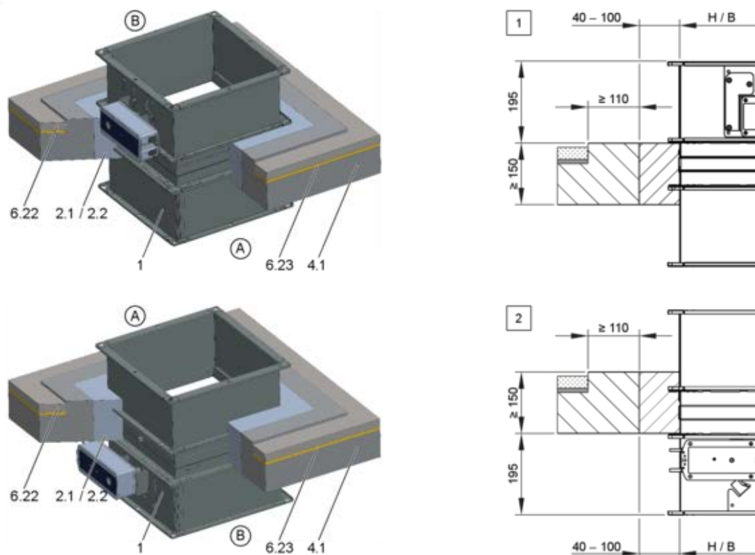
Fig. 29: Montagem em argamassa em tetos maciços com betonilha e isolamento acústico de passos, vertical e suspenso
