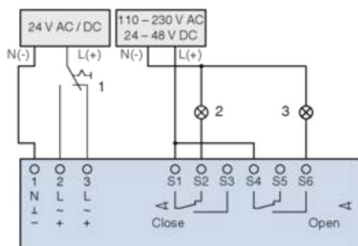
① Interruptor para abertura e fecho, a ser fornecido por terceiros ② Sinalizador luminoso para posição FECHADO, a ser fornecido por terceiros ③ Sinalizador luminoso para posição ABERTO, a ser fornecido por terceiros
