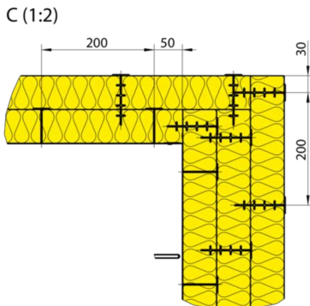
Fig. 78: EKA2-EU sobre conduta de extração de fumos em chapa de aço e isolamento térmico com material de isolamento térmico de 60 mm
