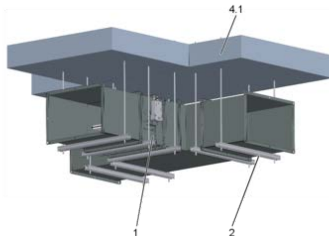
Fig. 46: Montagem ao lado de condutas horizontais de uma chapa de aço E600 120 (ved i ↔ o) S
