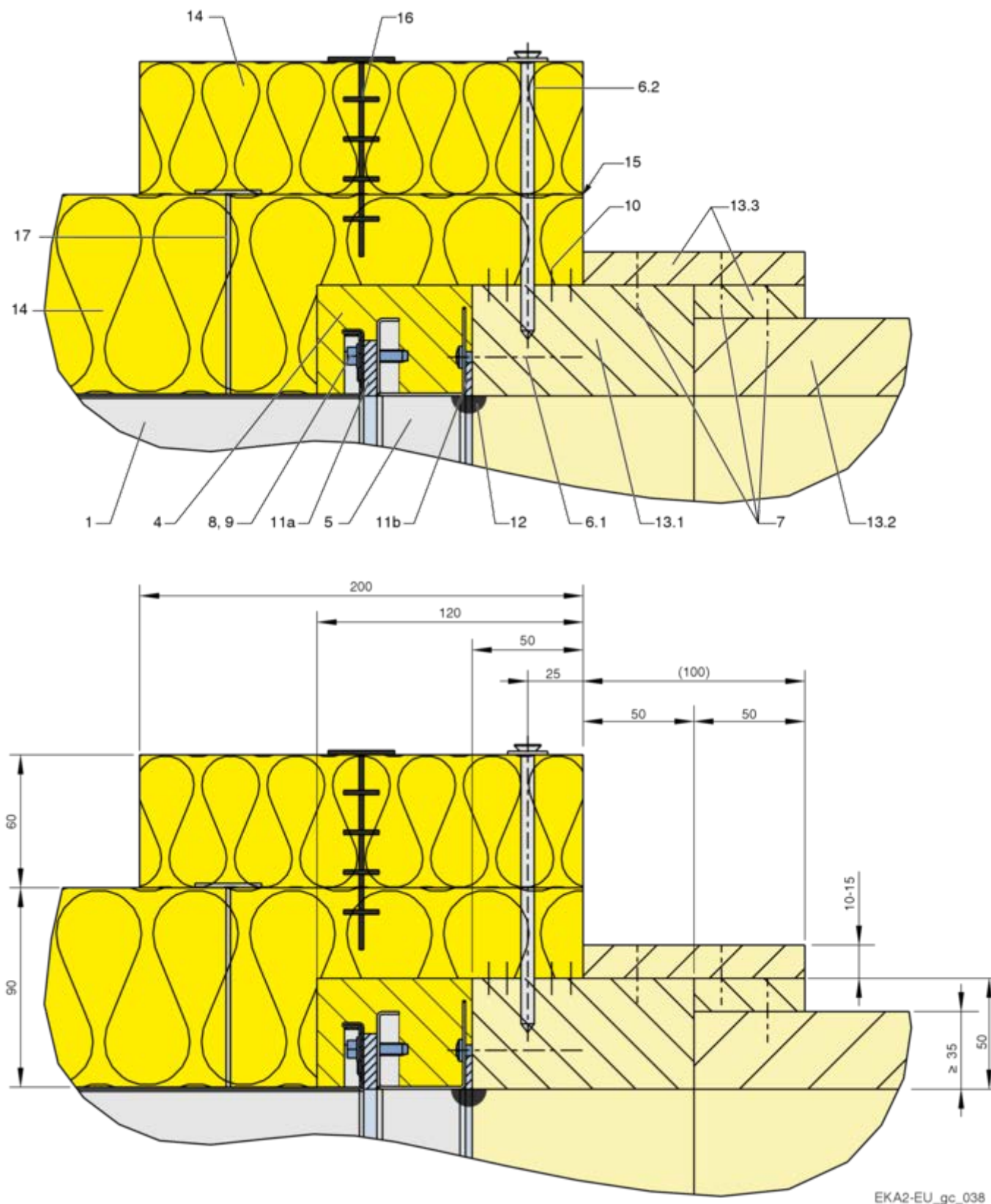
Fig. 79: Ligação da EKA2-EU - estrutura de ligação - conduta de extração de fumos de silicato de cálcio
