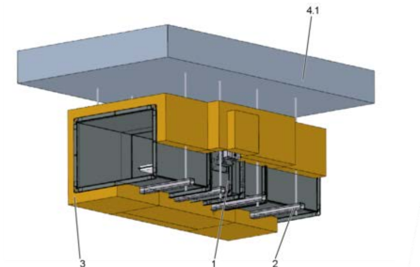
Fig. 40: Montagem em condutas horizontais de várias chapas de aço EI 120 ( _{ved} i \leftrightarrow o ) S
