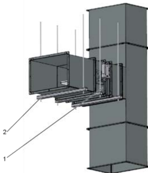
Fig. 47: Montagem ao lado de condutas horizontais de uma chapa de aço E600 120 ( v_{ed} i \leftrightarrow o ) S
