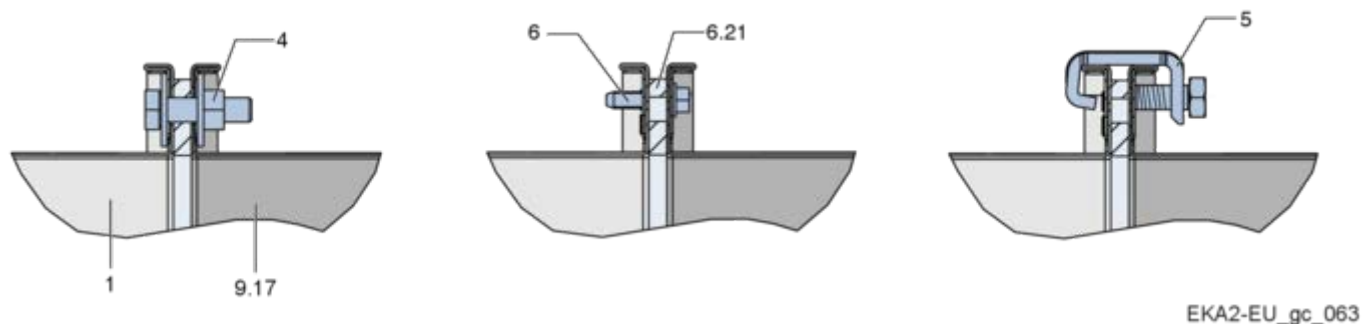
Fig. 76: EKA2-EU na conduta de extração de fumos em chapa de aço
