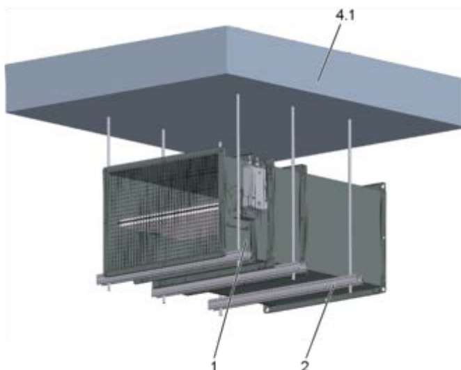
Fig. 45: Montagem na extremidade de condutas horizontais de uma chapa de aço E600 120 ( ved i ↔ o ) S
