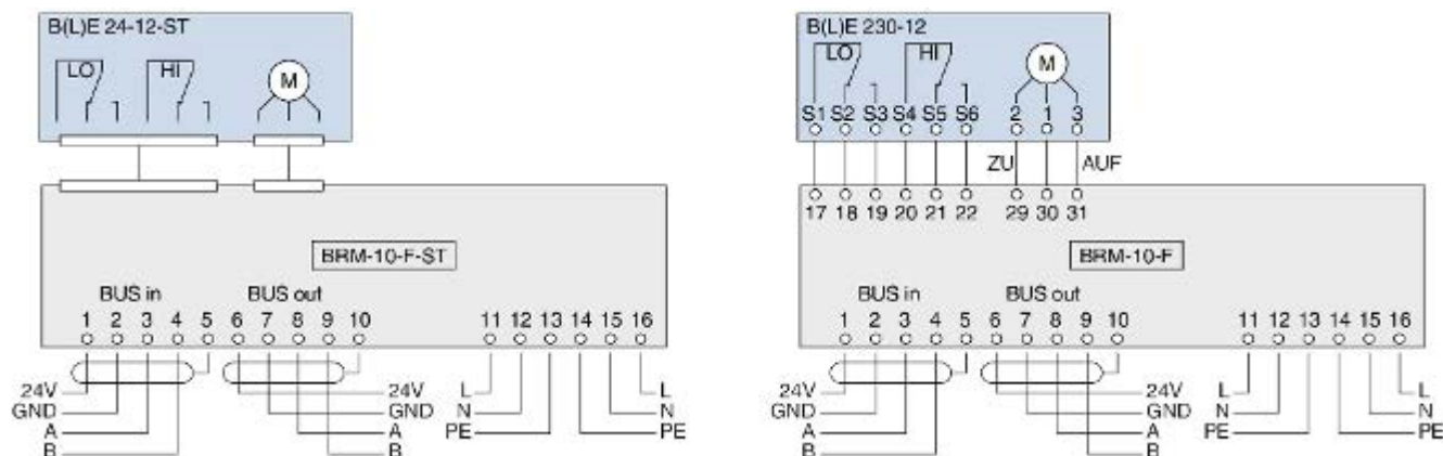
Fig. 83: Exemplo de cablagem para os anexos B24D e B230D
