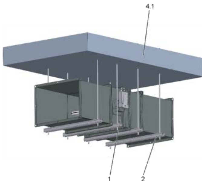
Fig. 44: Montagem em condutas horizontais de uma chapa de aço E600 120 ( _{ved} i \leftrightarrow o ) S
