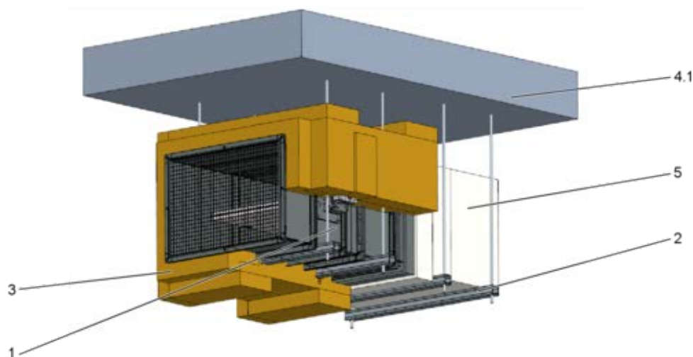
Fig. 38: Montagem na extremidade de condutas horizontais independentes de extração de fumo EI 120 ( ved i ↔ o ) S
