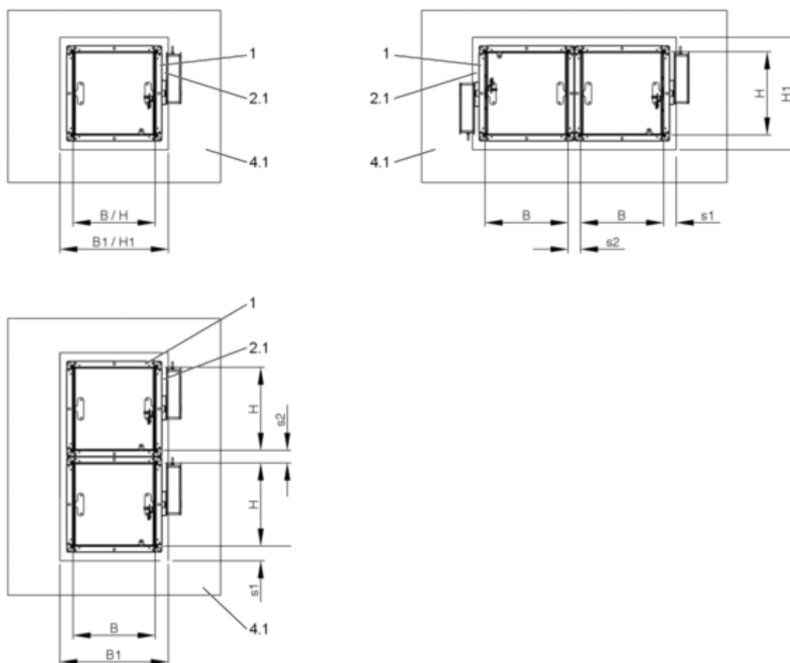
Fig. 26: Placas de teto maciças – disposição/distâncias
